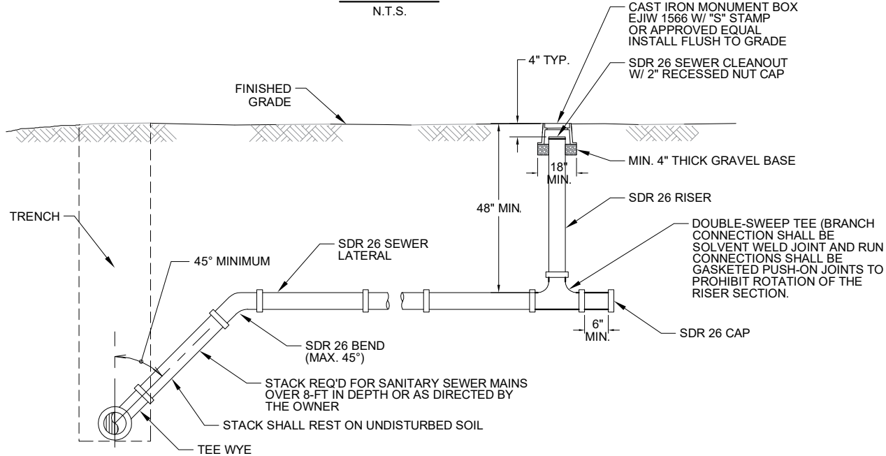
ELEVATION VIEW N.T.S.
